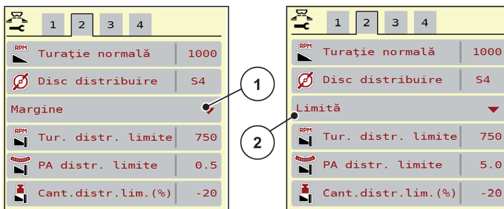
Fig. 14: Valori de setat Mod împrăștiere limitată
