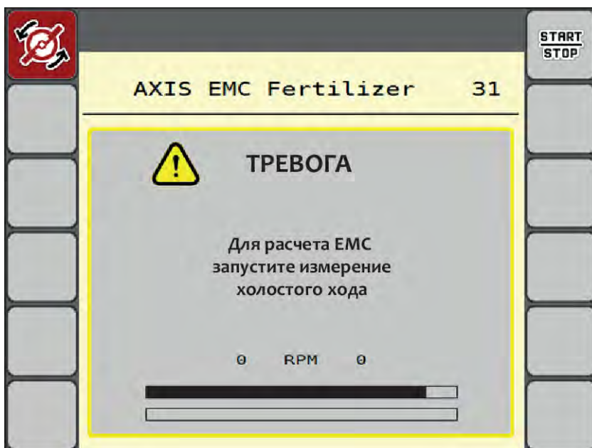
Рис. 43: Аварийная индикация измерения холостого хода
