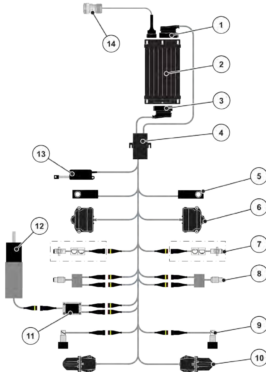
Фиг. 6: AXIS-H EMC: Схематичен изглед на свързването
