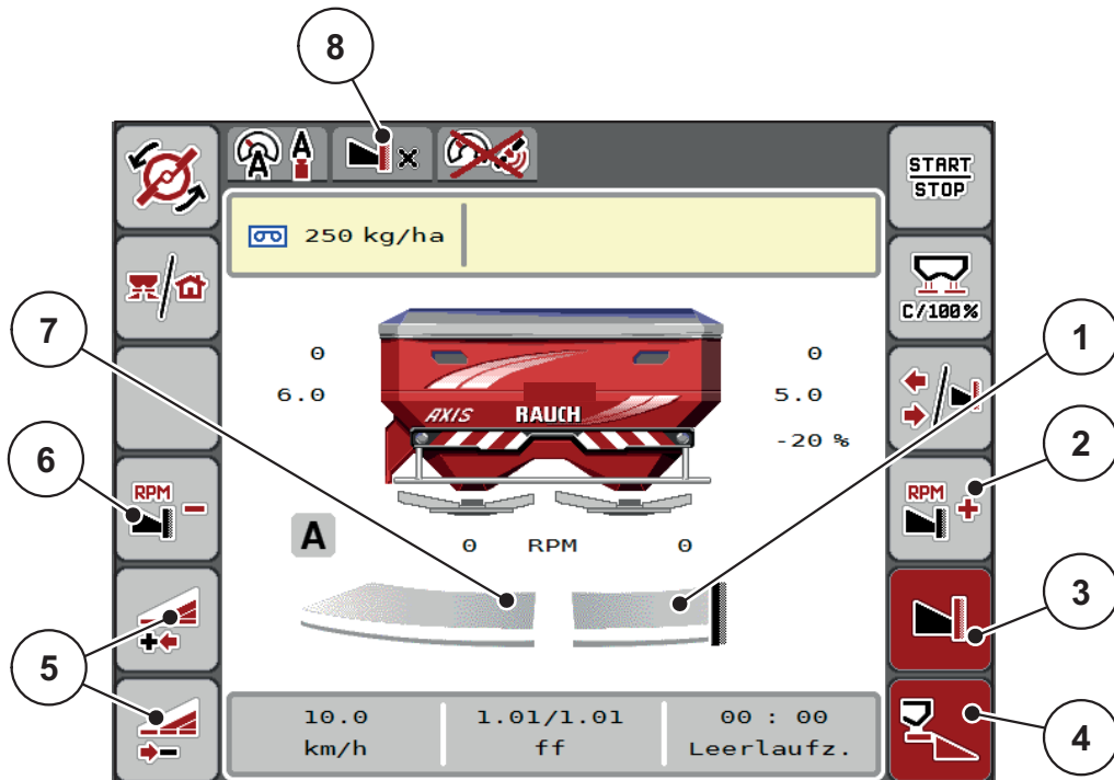
5.5 ábra: Üzemi képernyő: részszélesség a bal oldalon, határszórás a jobb oldalon
