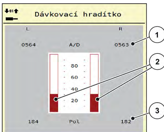
Obr. 23: Test/diagnostika; Příklad: Dávkovací hradítko
