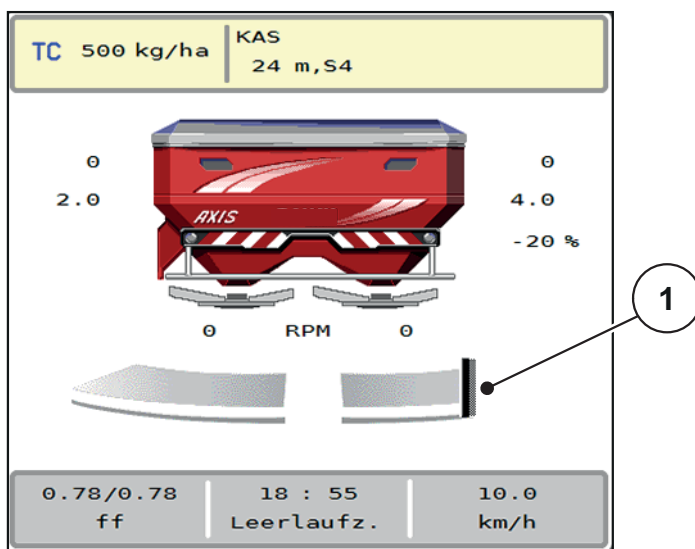
Afb. 5.2: Weergave TELIMAT
