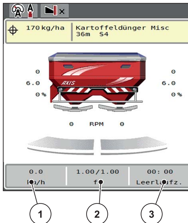
Afb. 2.3: Weergavevelden
