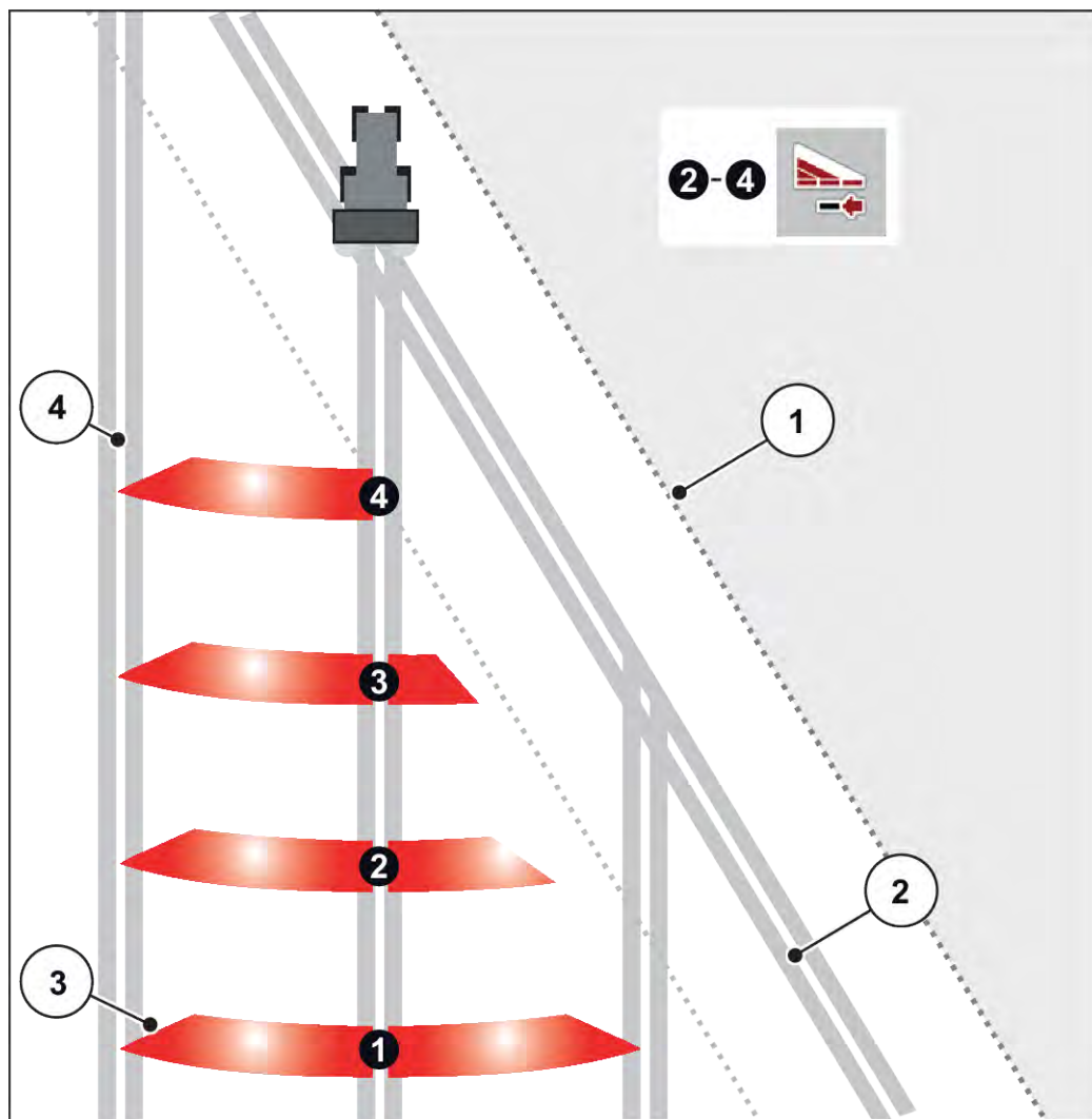
Abb. 39: Automatische Teilbreitenschaltung
