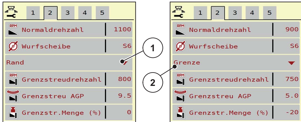
Bild 4.6: Einstellwerte Grenzstreumodus
