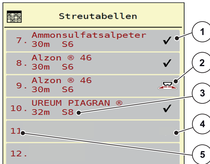
Bild 4.9: Menü Streutabellen
