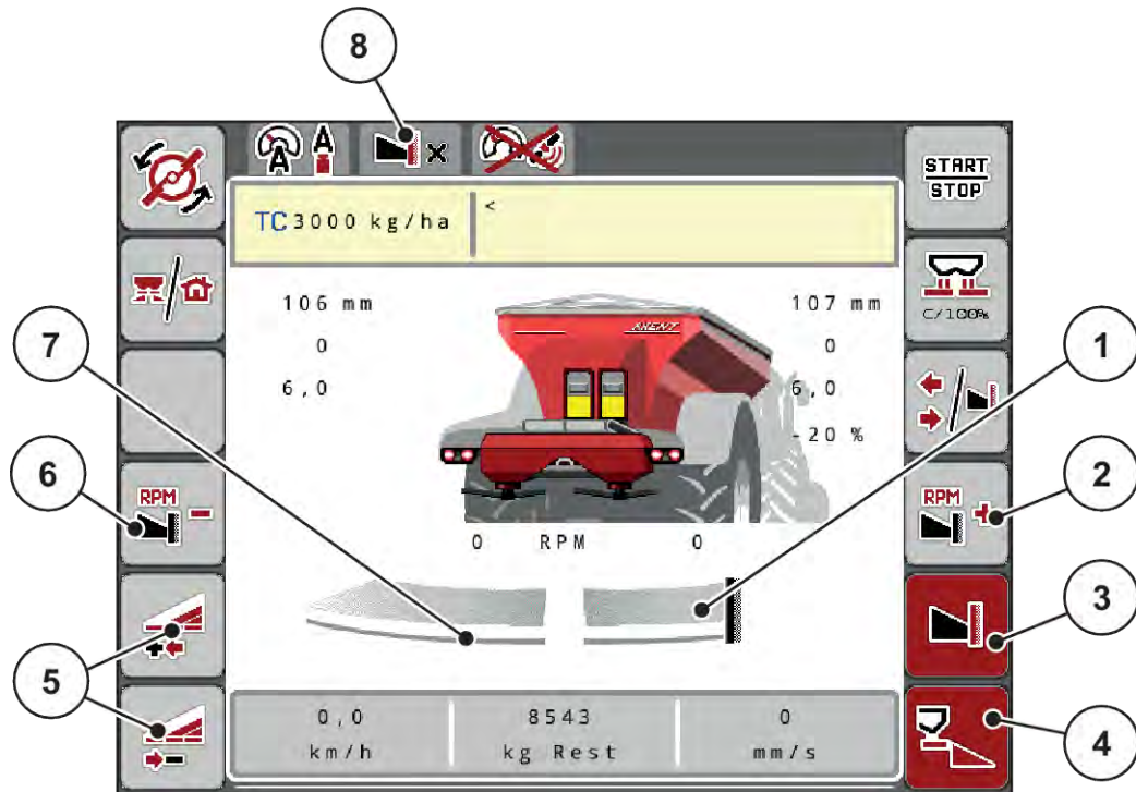
Ilust. 39: Pantalla de funcionamiento de una anchura parcial izquierda, lado de dispersión límite derecho
