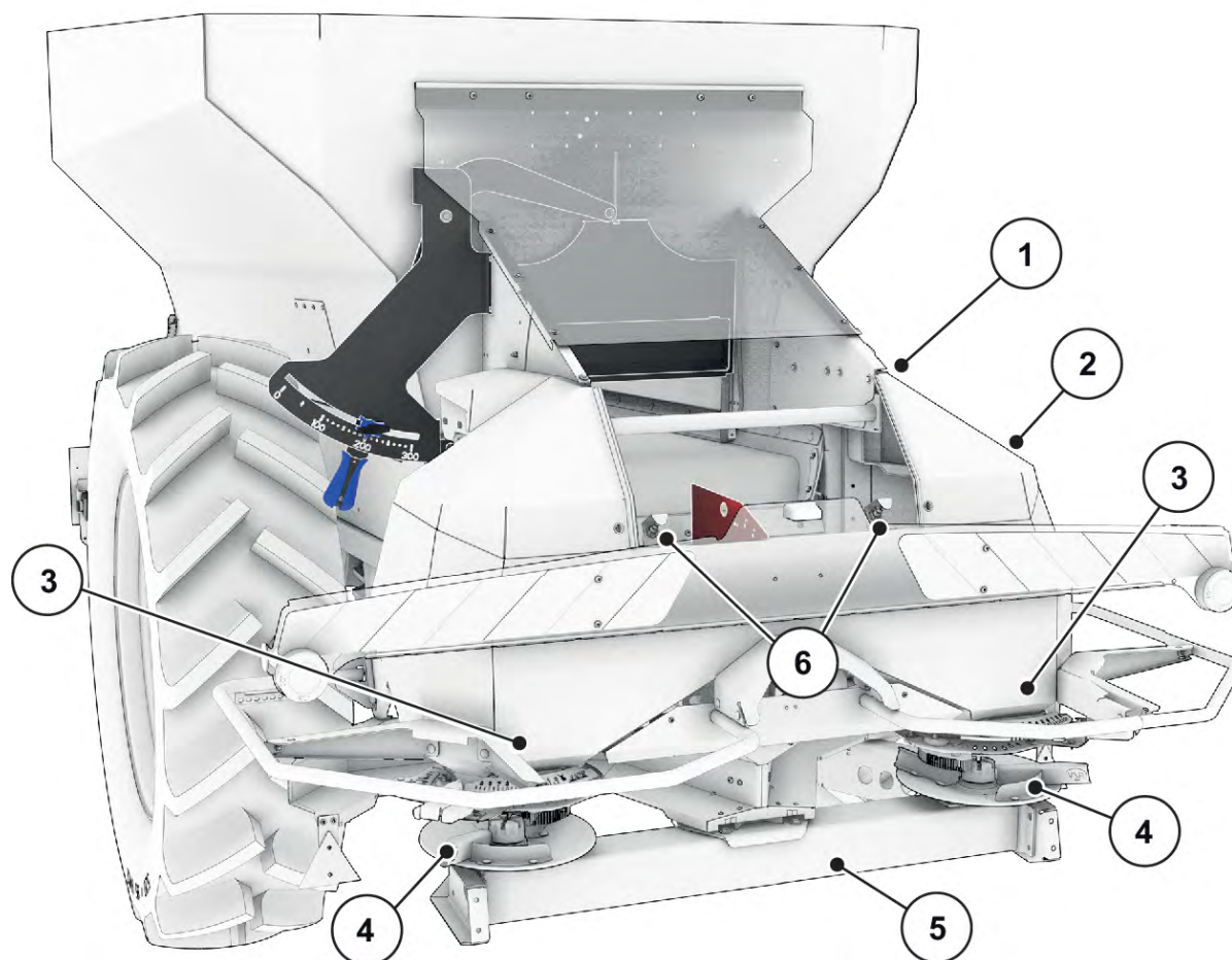
Ilust. 6: Vista general de los actuadores y sensores en la abonadora de gran superficie AXENT y el mecanismo de dispersión de fertilizante
