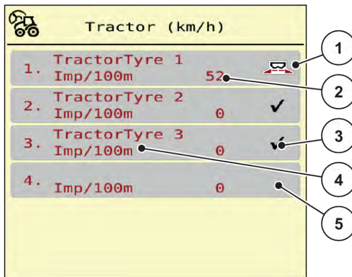
Ilust. 20: Menú Tractor (km/h)
