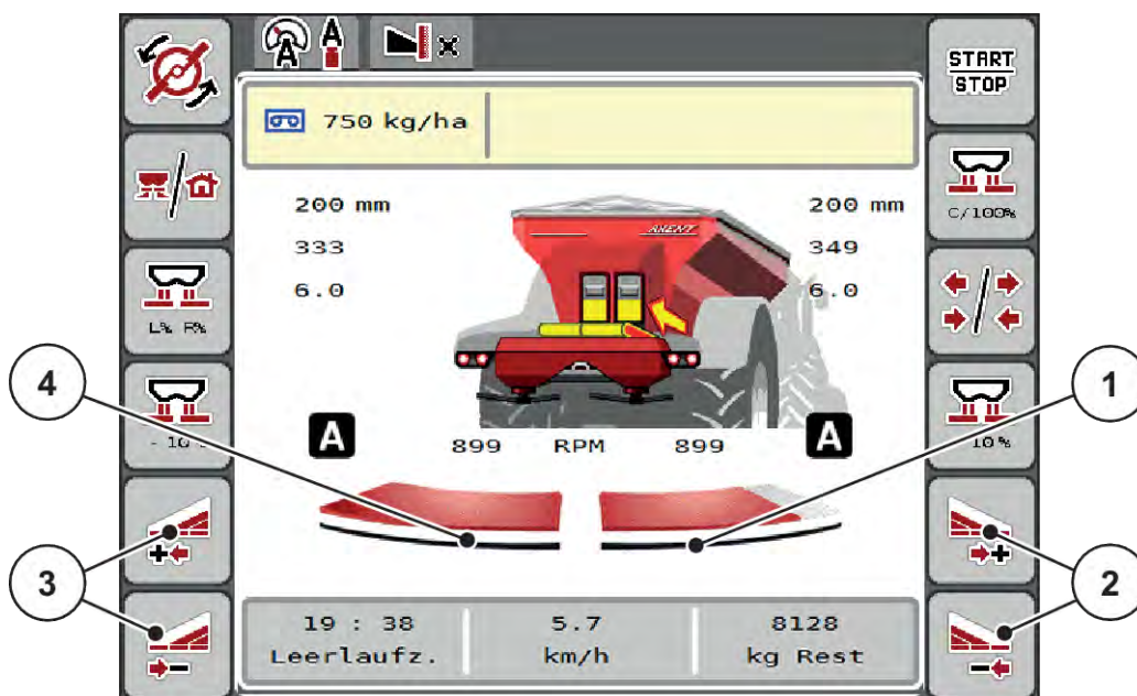
Ilust. 37: Pantalla de funcionamiento: Anchuras parciales con 2 niveles
