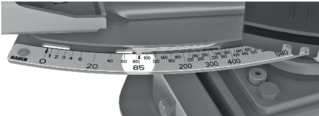
Kuva 68: Asteikko levitysmäärän näyttöön
