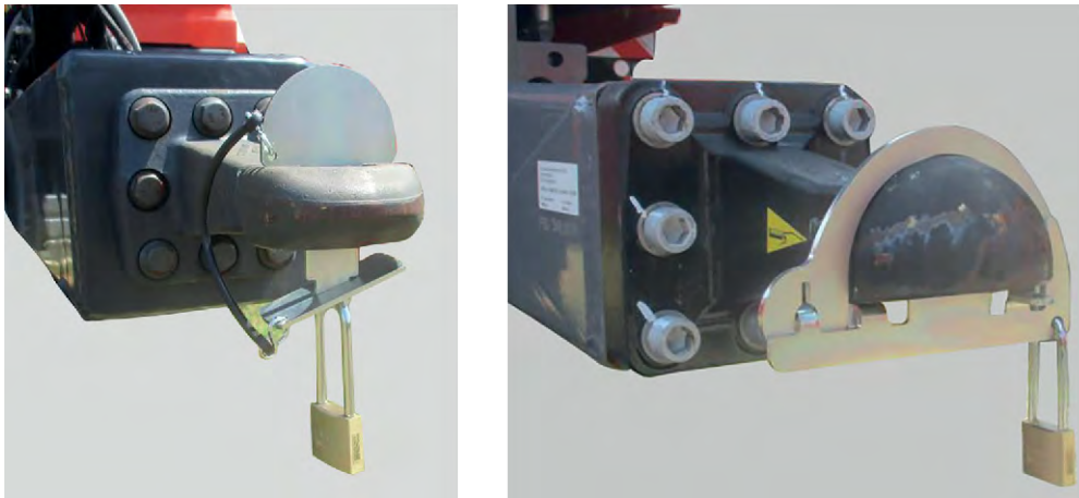
Kuva 12: Vetolaitteen käytönestojärjestely
