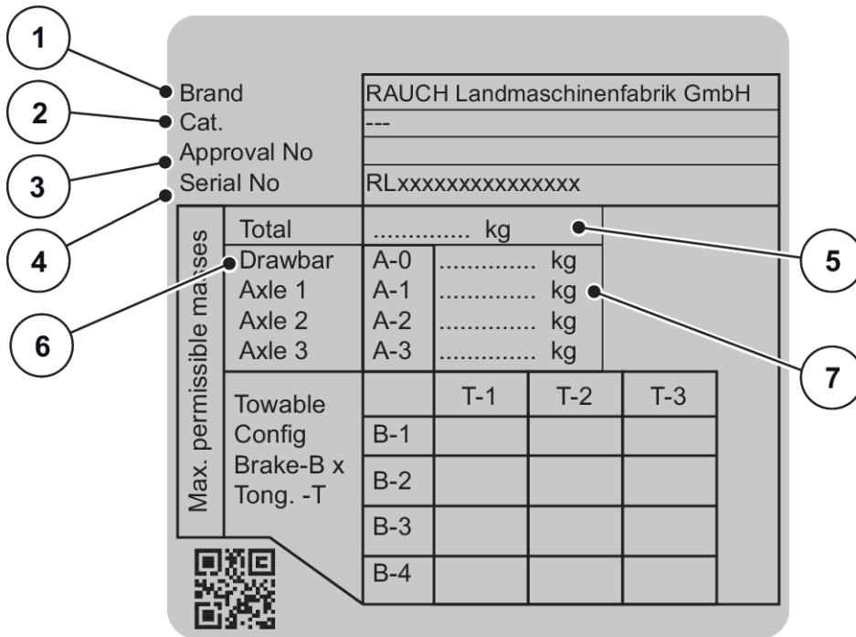
Kuva 8: Luokittelukilpi
