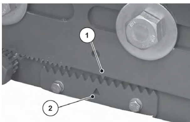
Kuva 73: Luovutus piste vapaa-asennossa
