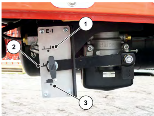
Kuva 30: Jarruvoimasäätimen asettaminen
