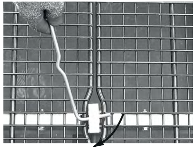
Kuva 40: Suojaritilän lukitseminen
