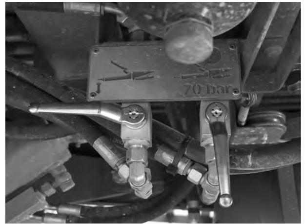
Kuva 113: Vasemman sulkuventtiilin sulkeminen
