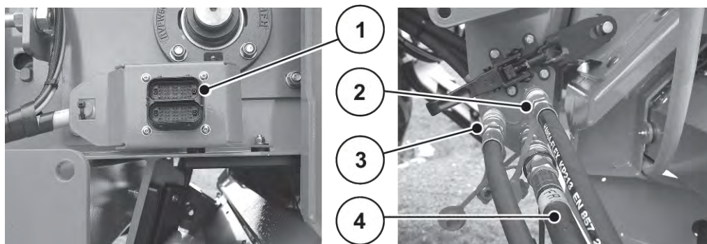
Kuva 45: Liitännät
