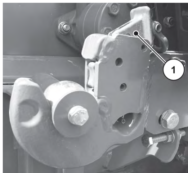
Kuva 48: KytKentäpisteiden irrotus
