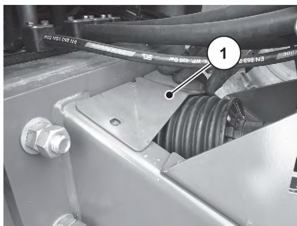
Kuva 23: Suojalevyn asennus
