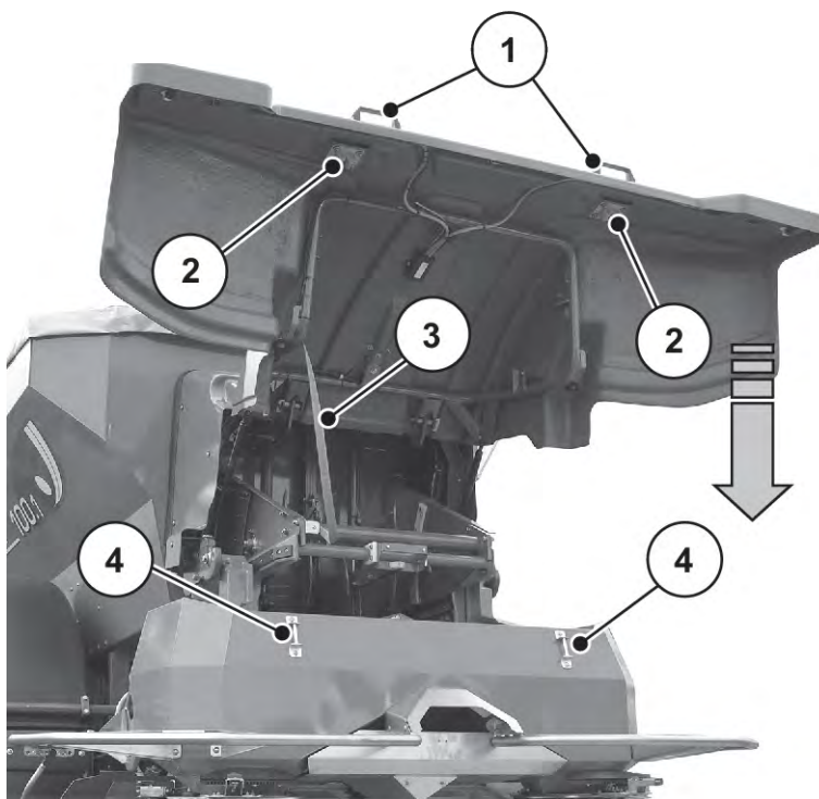
Kuva 58: Suojakannen osat
