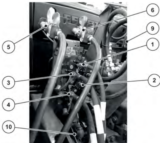
Kuva 25: Konelinjojen liitäntäjärjestys traktoriin
