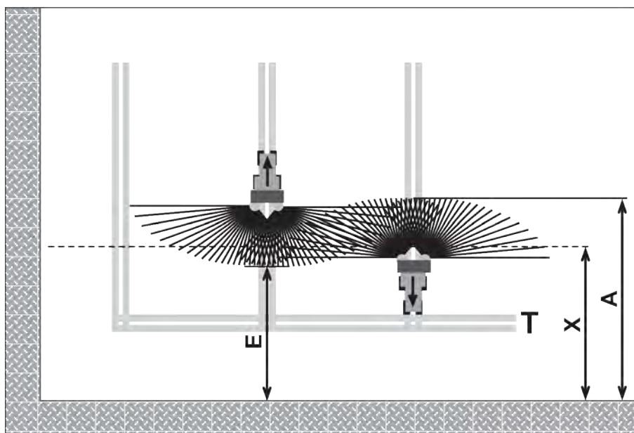
Kuva 70: Normaalilevitys
