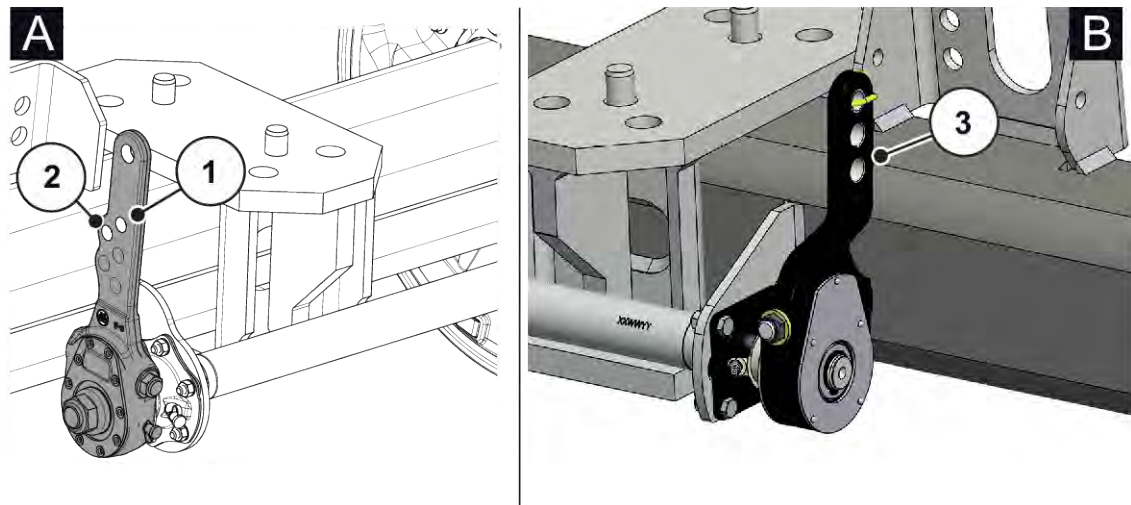
Kuva 129: Jarruvivun/jarrusylinterin liitännän sijainti – jäykkä akseli
