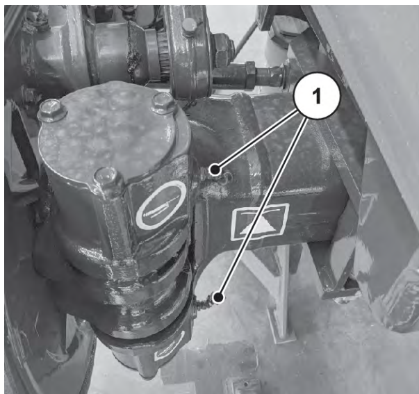
Kuva 96: Ohjaava akseli
