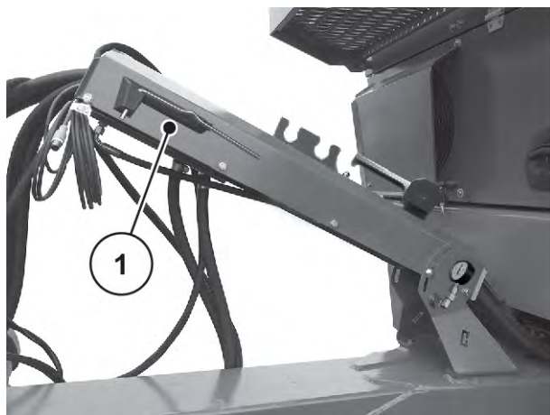
Kuva 32: Asetusvivun paikka
