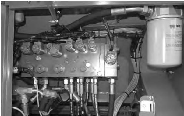
Kuva 100: Ohjauslohko
