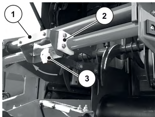
Kuva 37: Erotuslevyn varmistaminen
