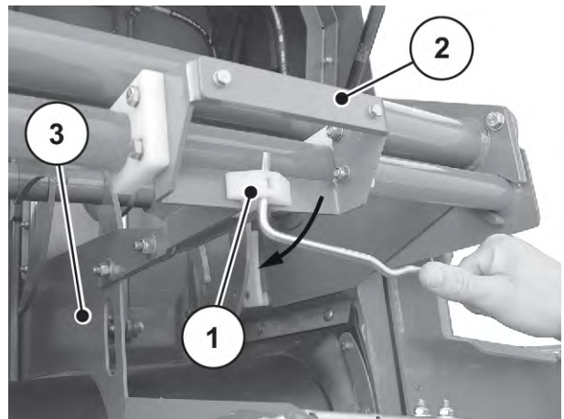
Kuva 34: Irrota erotuslevy.
