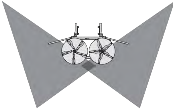
Kuva 75: Liian vähän lannoitetta tai kalkkia keskellä
