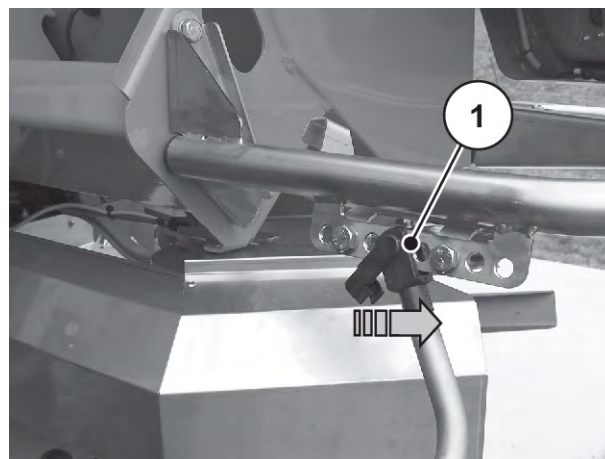
Kuva 46: Lokasuojan jatkeen kiinnittäminen
