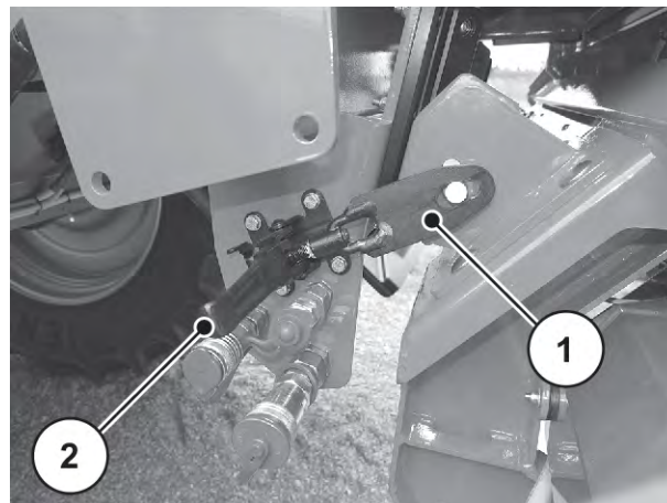
Kuva 44: Levittimen varmistaminen alhaalta
