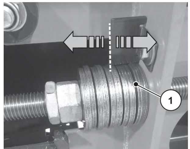
Kuva 120: Levyjousipakettien asetus
