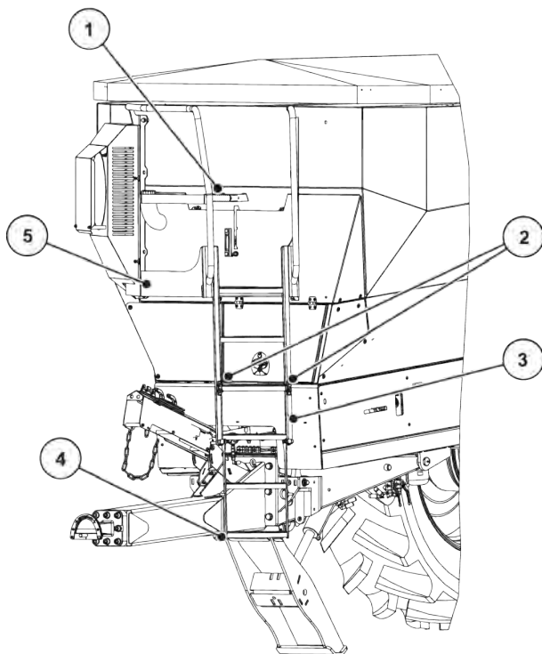
Kuva 51: Täyttötason tarkistus
