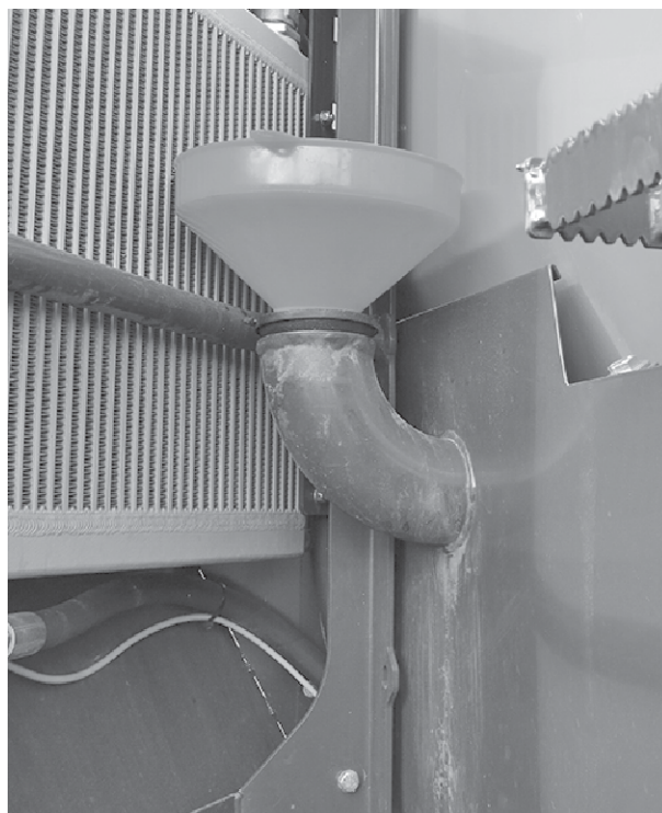
Kuva 106: Öljyn täyttö
