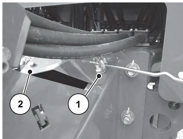
Kuva 20: Suojalevyn irrotus
