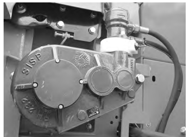
Kuva 103: Kuljetinhihnamoottorin tarkistus
