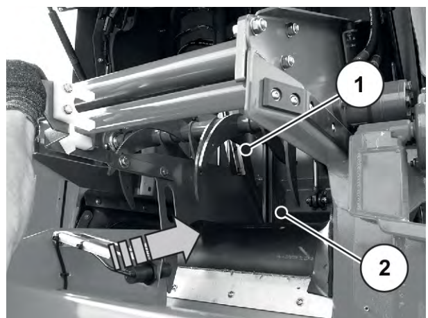
Kuva 35: Erotuslevyn asennus
