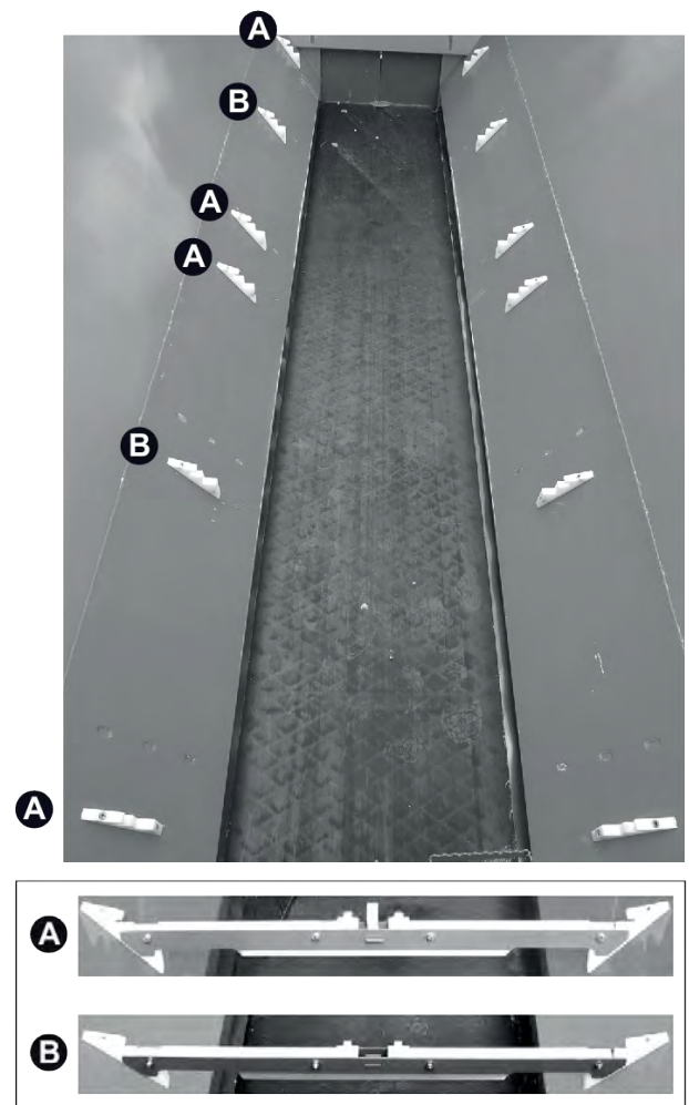
Kuva 38: Suojaritilän pidikkeiden asennus
