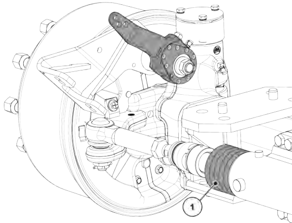
Kuva 107: Ohjauksakselin välilevyt
