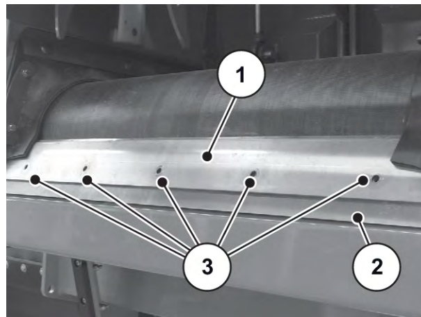
Kuva 121: Kiristyslevyn irrotus
