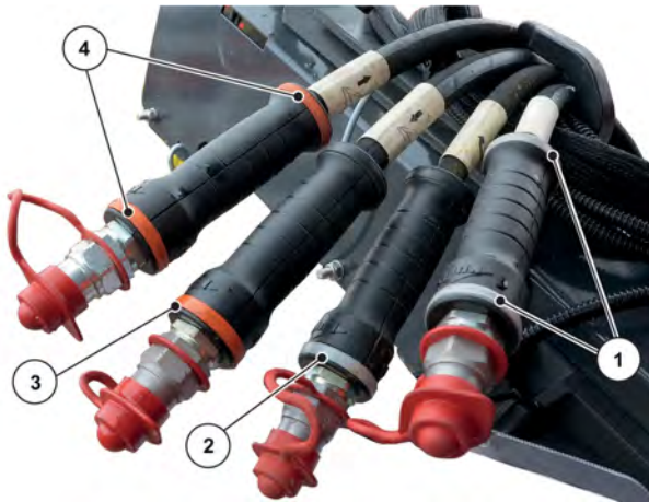
Kuva 26: Hydrauliletkujen tunnistus
