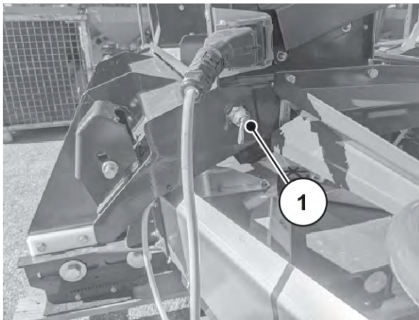
Kuva 97: Voitelukohta, yleislevitin
