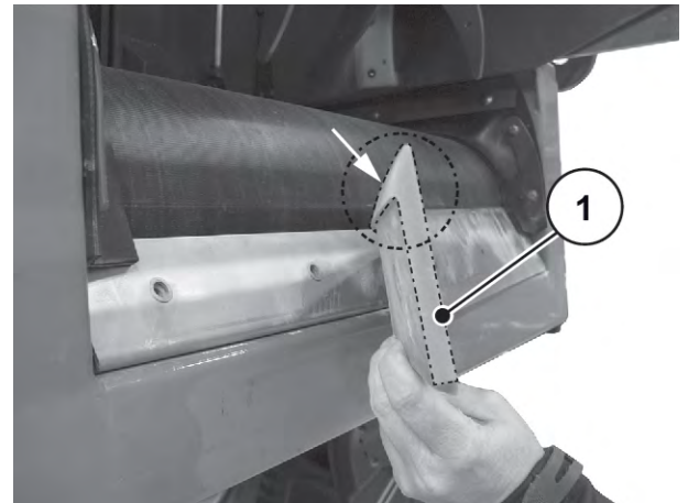
Kuva 124: Kiristyslevyn asettaminen paikalleen
