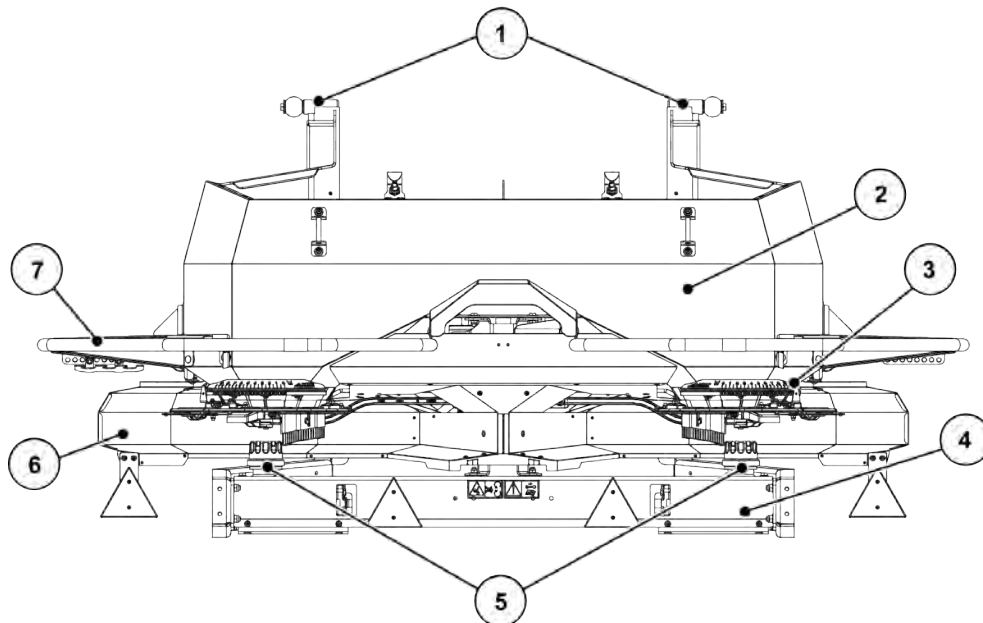
Kuva 13: AXIS-PowerPack-lannoitelevittimen rakenneryhmäkuva
