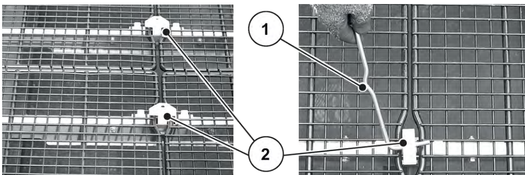
Kuva 33: Pidikkeiden vapauttaminen
