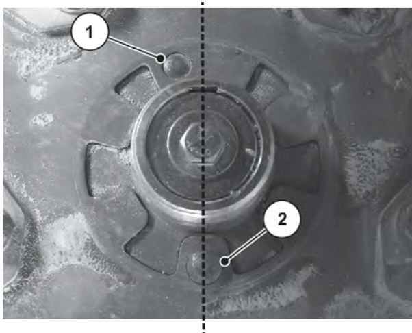
Kuva 110: Levityslautasten eri puolet ovat erilaisia
