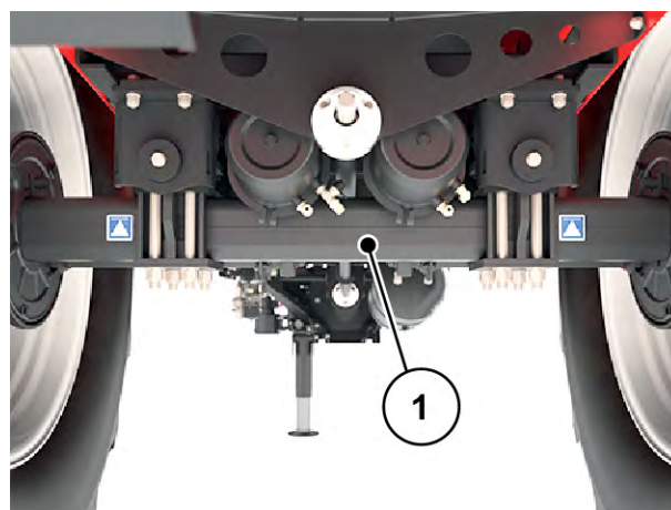
Kuva 131: Koneen hätähinaus köyden avulla
