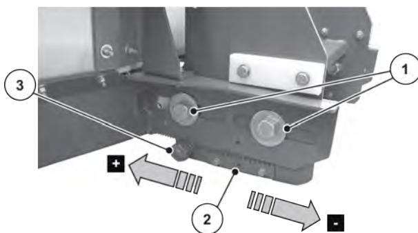
Kuva 74: Luovutus pisteen asettaminen
