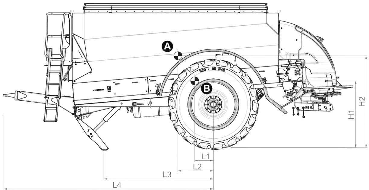
Kuva 16: Painopiste yläripustuksessa
