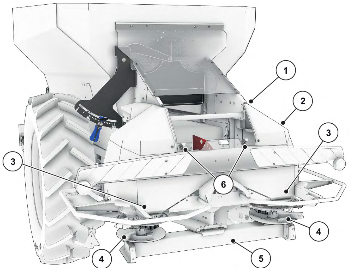
Abb. 6: Übersicht der Aktoren und Sensoren am Großflächenstreuer AXENT und Düngerstreuwerk
