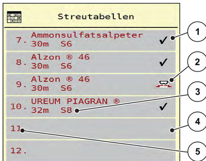
Abb. 15: Menü Streutabellen
