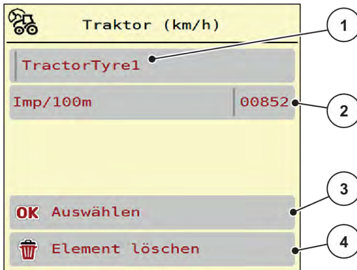
Abb. 21: Traktorprofil
