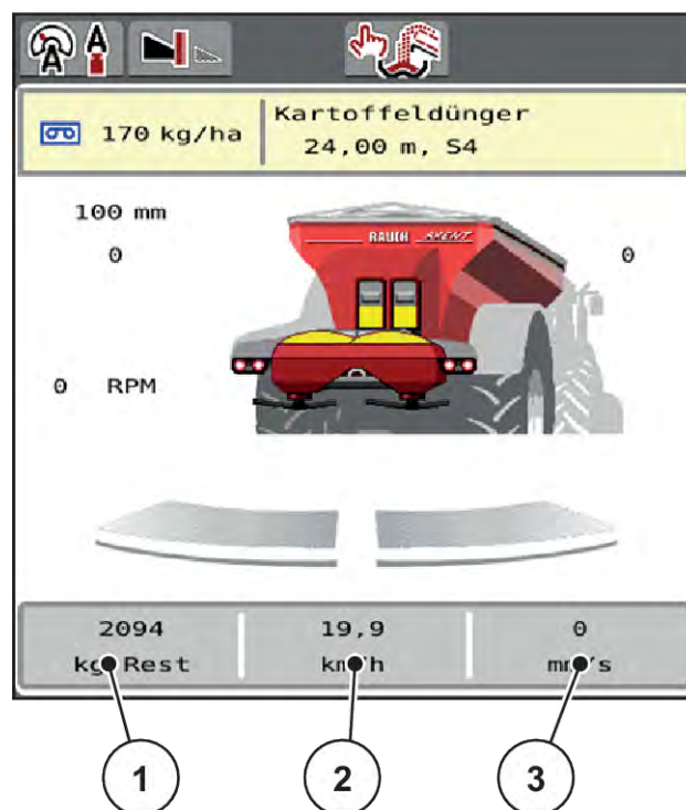
Abb. 2: Anzeigefelder
