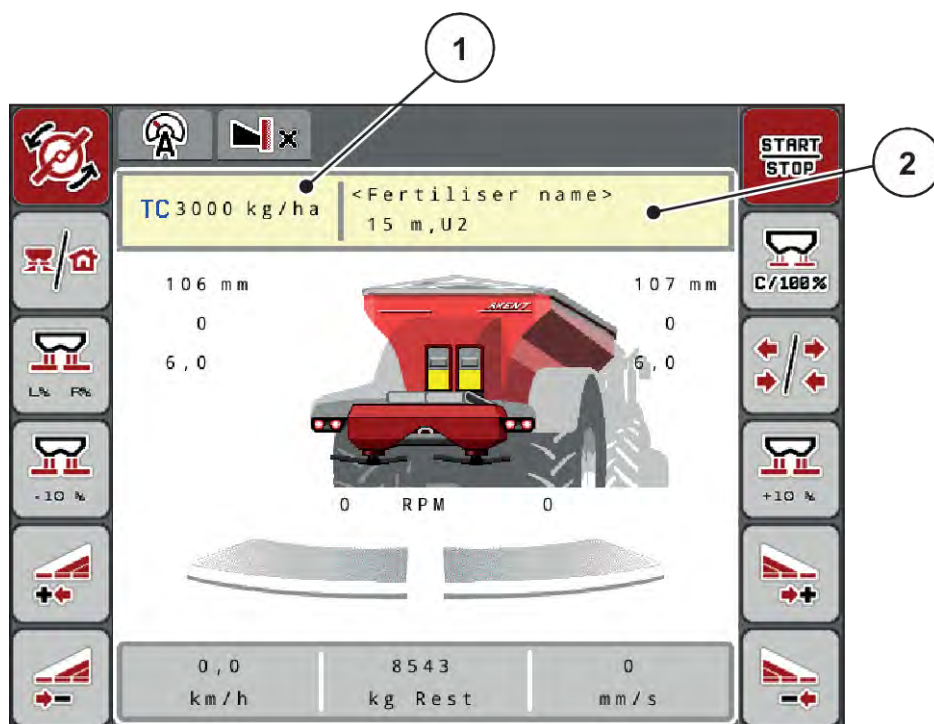
Fig. 12: Saisie de la dose sur l'écran tactile
