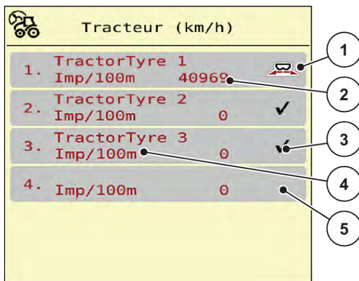
Fig. 24: Menu Tracteur (km/h)
