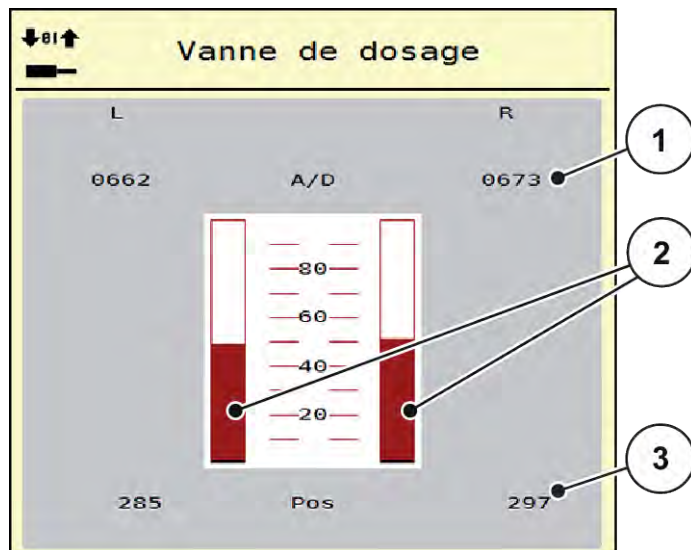
Fig. 31: Tests/Diagnostic ; exemple : Vanne de dosage
