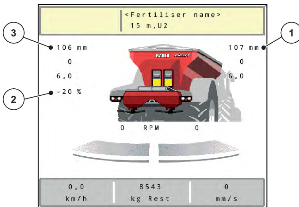
Fig. 48: Écran de travail Secteur MAN
