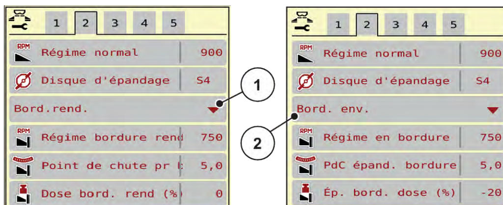
Fig. 13: Valeurs de réglage mode d'épandage en bordure
