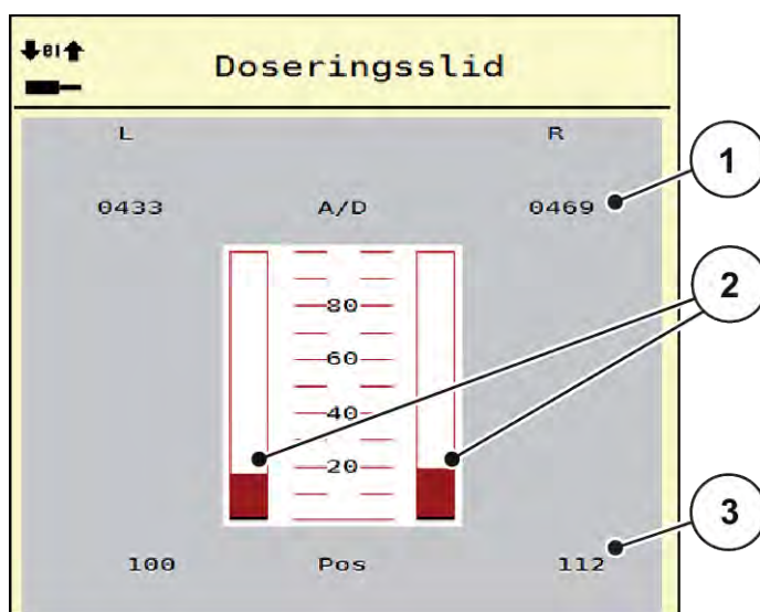
Fig. 31: Test/diagnos; Exempel: Doseringsslid
