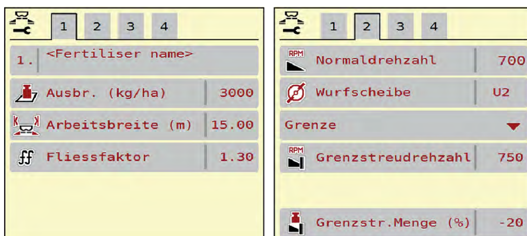
Fig. 18: Meny Gödselinst., kalkdrift flik 1 och 2
