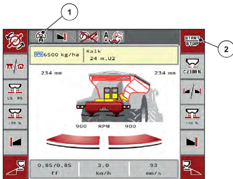
Fig. 52: Driftbild i kalkdrift
