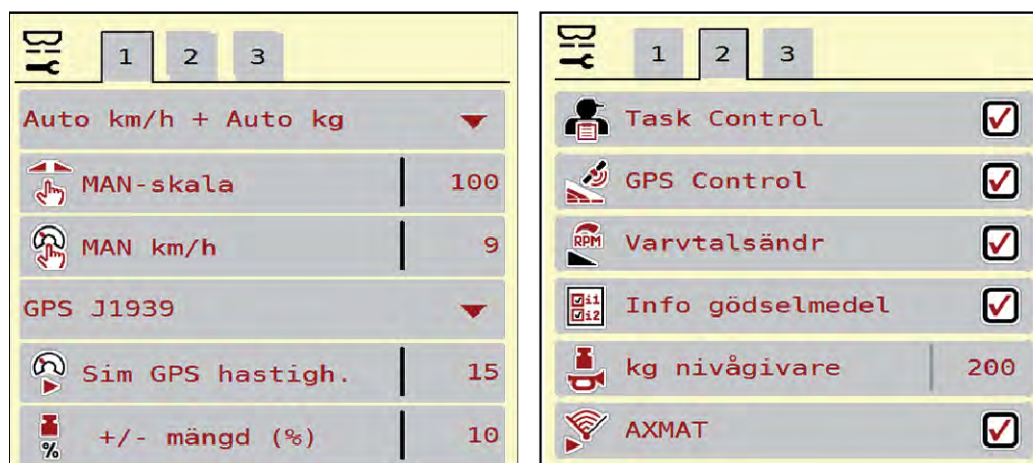
Fig. 20: Meny Maskininställningar, flik 1 och 2
