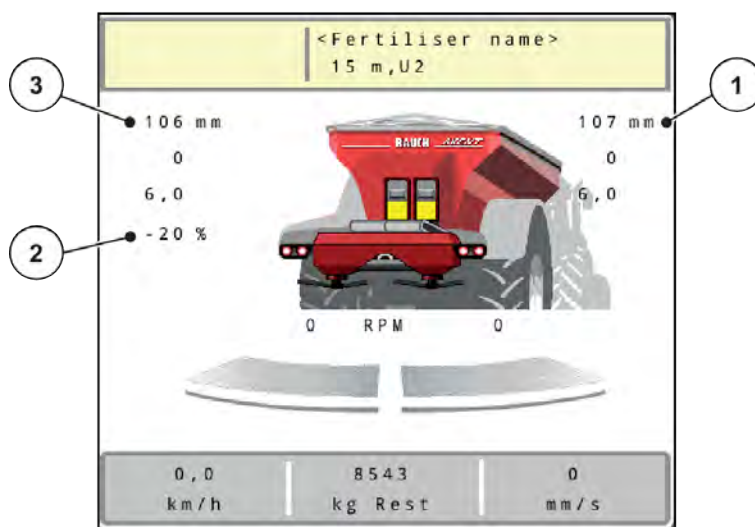
Fig. 48: Driftsbild MAN-skala
