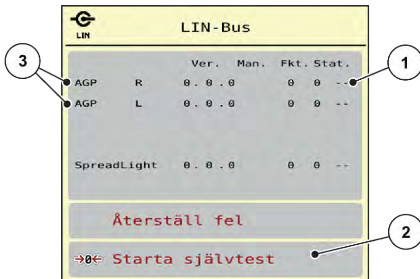
Fig. 32: System/test; Exempel: Test/diagnos
