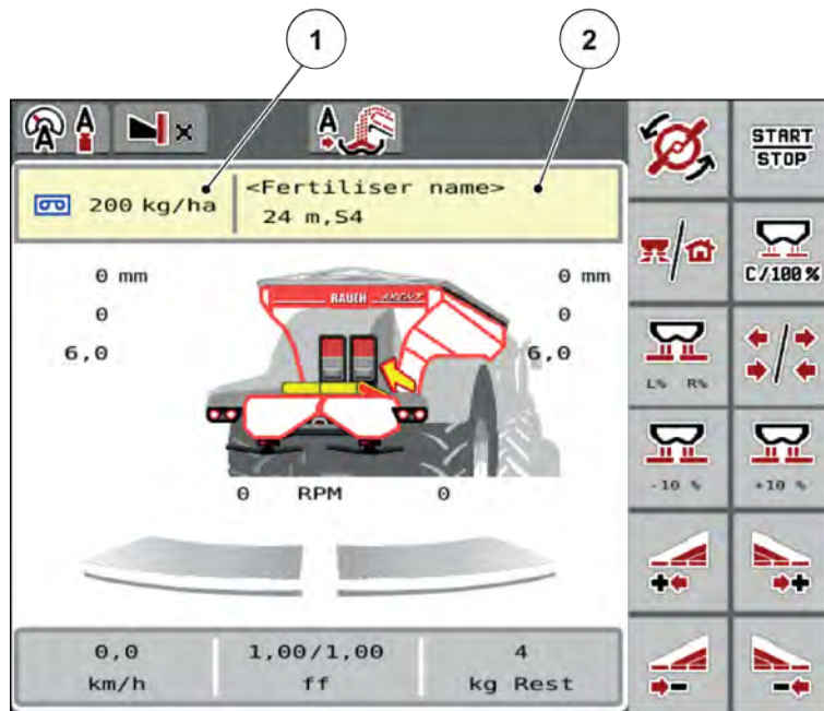
Fig. 17: Hantera spridningstabellen på pekskärmen
