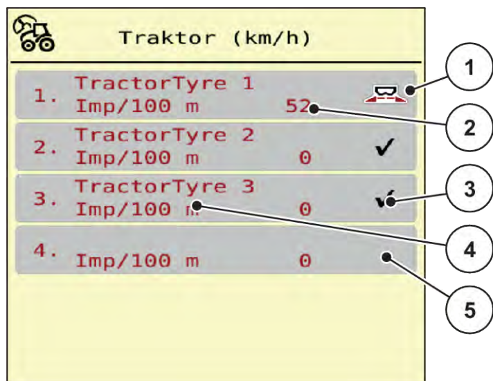
Ábr. 24: Menü Traktor (km/h)
