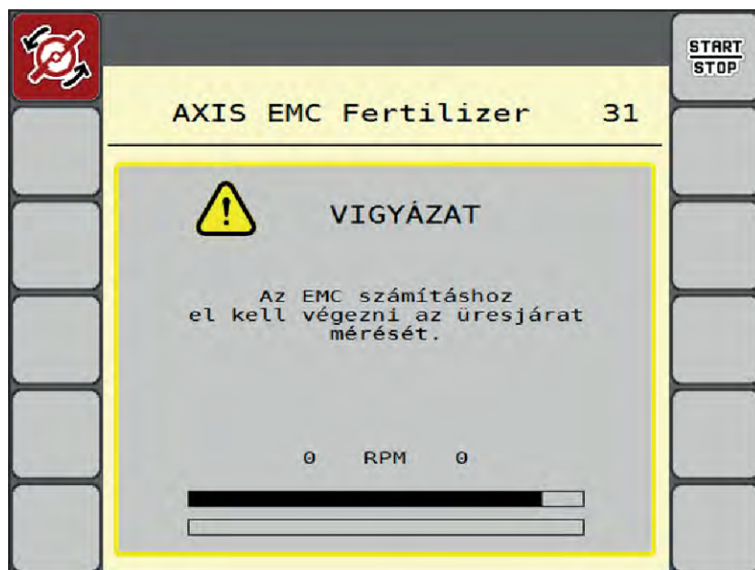
Ábr. 46: Az üresjárat mérés riasztásjelzése
