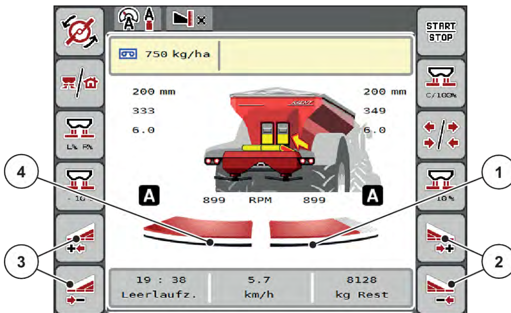
Ábr. 43: Üzemi képernyő: Részszelességek 2 részszelességgel
