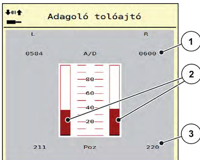
Ábr. 31: Teszt/diagnózis; példa: Adagoló tolóajtó
