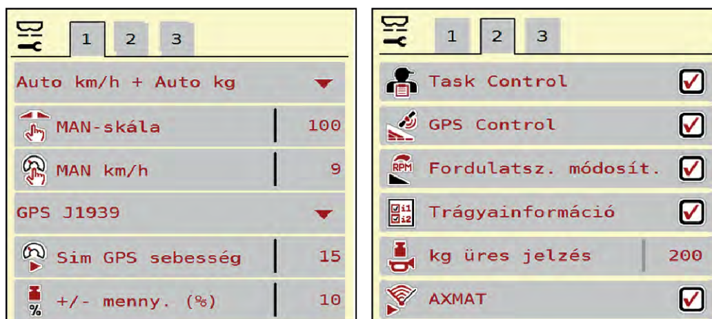
Ábr. 20: Gépheállítások menü, 1. és 2. fül
