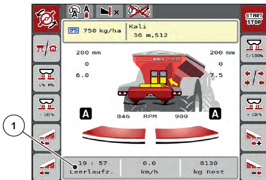
Pav. 49: Barstymo režimo rodmuo darbiniam lange su „GPS Control“
