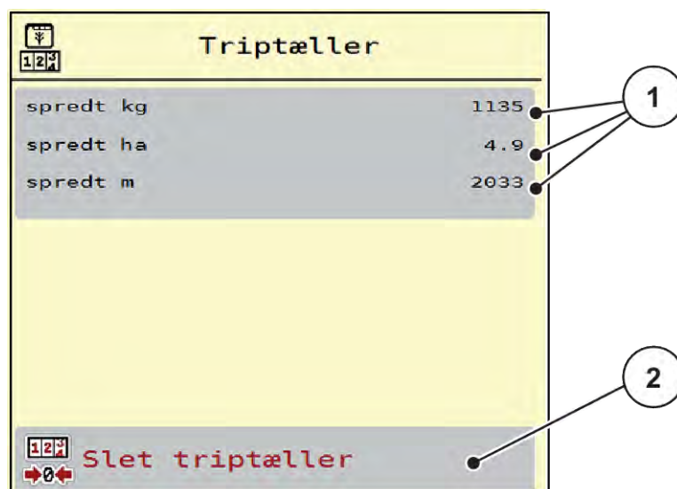
Fig. 34: Menu Triptæller
