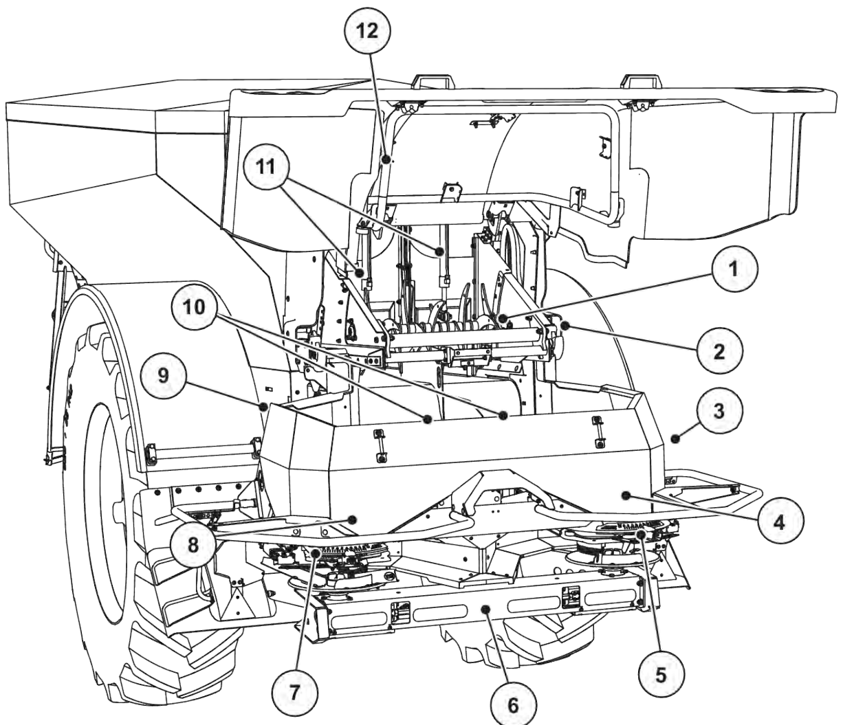
Fig. 6: Oversigt over aktuatorer og sensorer på spredemaskinen AXENT og gødningsspredværket AXIS-PowerPack
