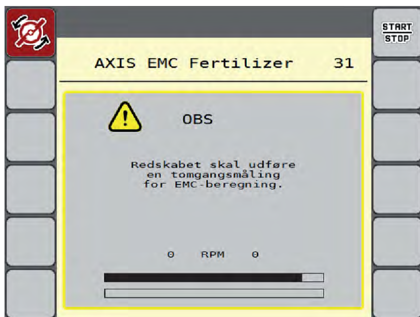
Fig. 46: Alarmvisning tomgangsmåling
