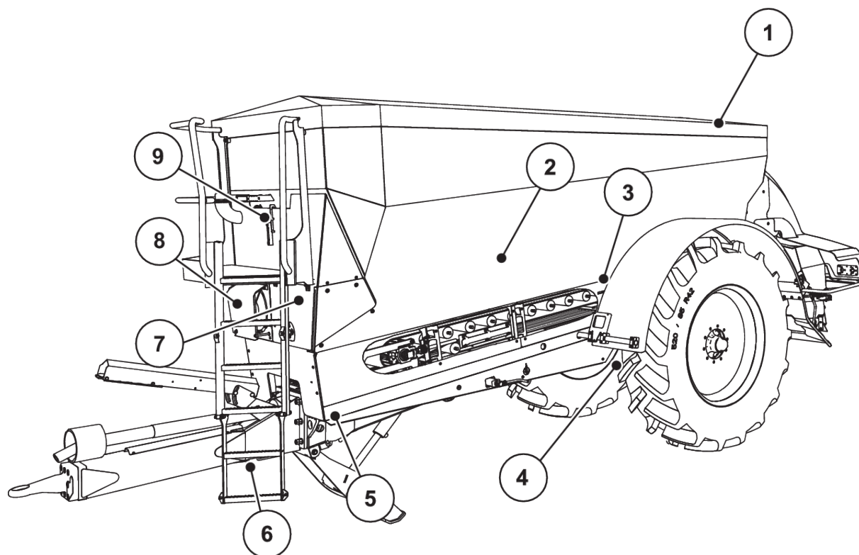
Rys. 5: Przegląd elementów wykonawczych i czujników w rozsiewaczu wielkopowierzchniowym AXENT
