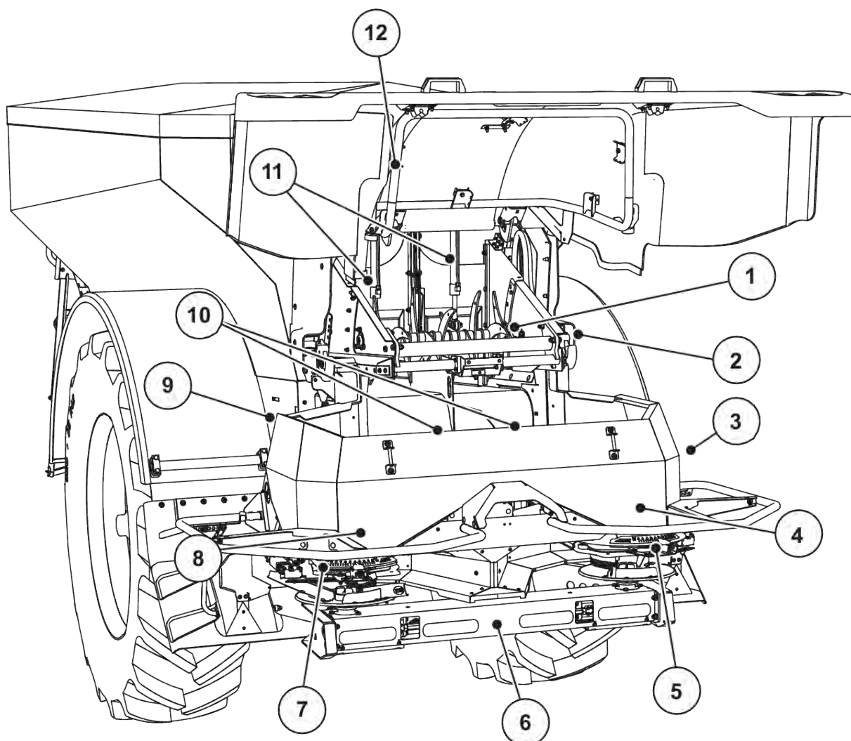
Rys. 6: Przegląd urządzeń wykonawczych i czujników w rozrzutniku wielkopowierzchniowym AXENT i rozrzutniku nawozu AXIS-PowerPack
