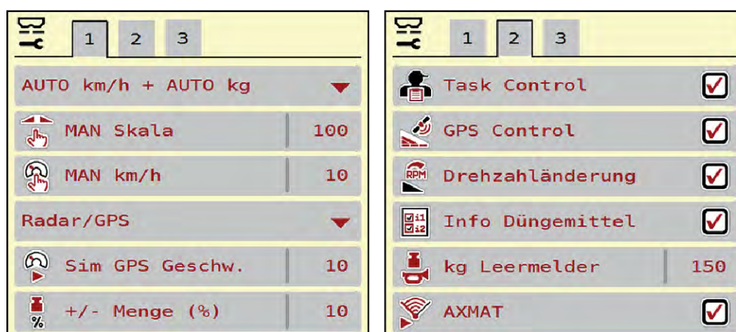
Abb. 20: Menü Masch. Einstellungen, Reiter 1 und 2
