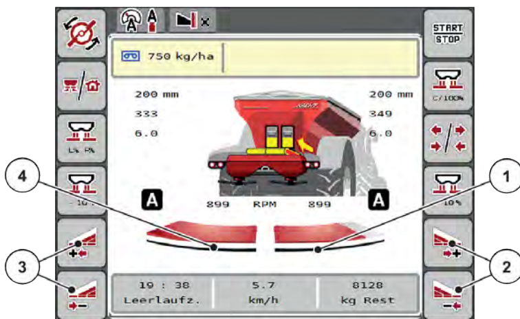
Abb. 43: Betriebsbild: Teilbreiten mit 2 Teilbreiten
