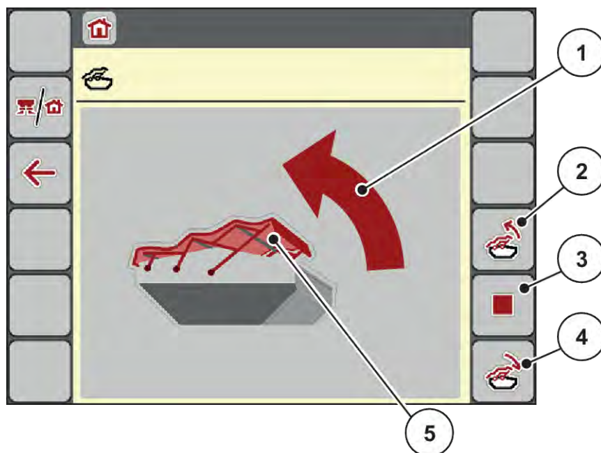
Fig. 26: Meniul Prelată
