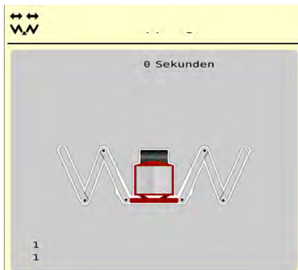
Fig. 13: Meniu Pliere
