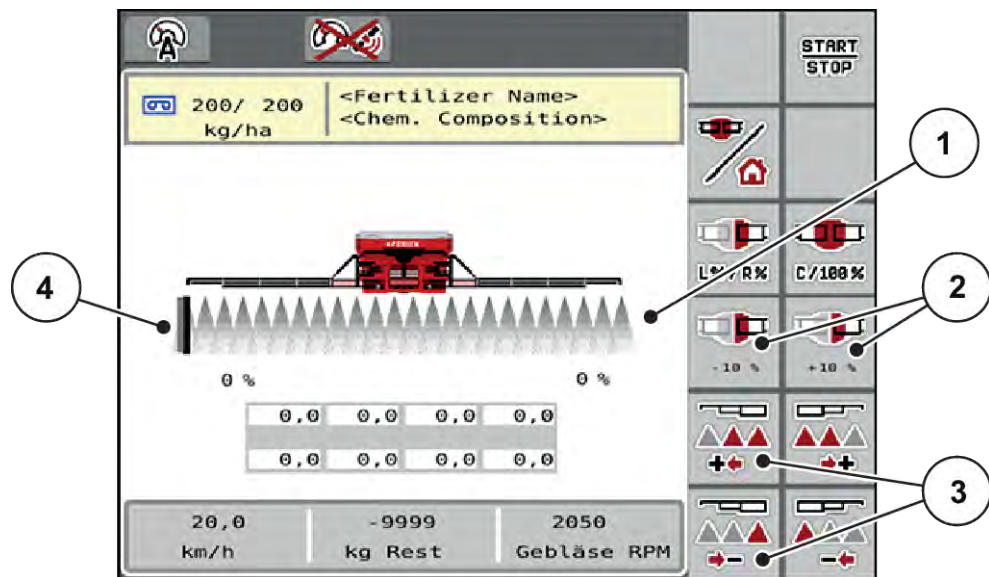
Fig. 32: Ecran de operare lățimi parțiale activate, împrăștiere la limită stânga
