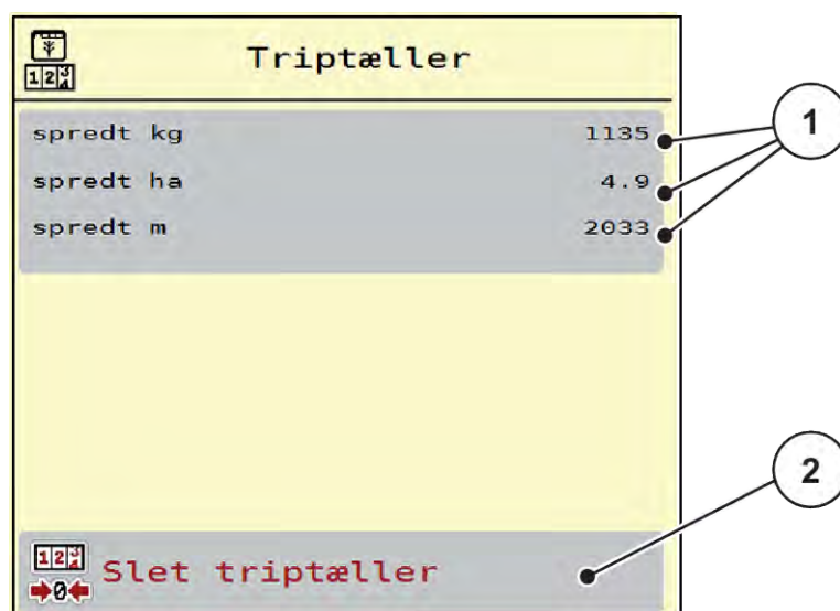
Fig. 21: Menu Triptæller
