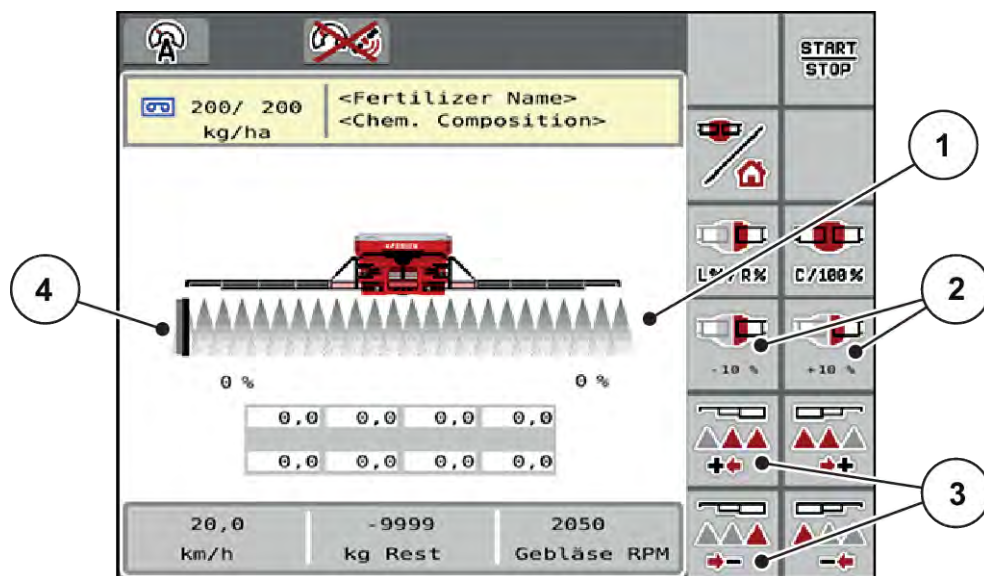
Abb. 32: Betriebsbild aktivierte Teilbreiten, Grenzstreuen links
